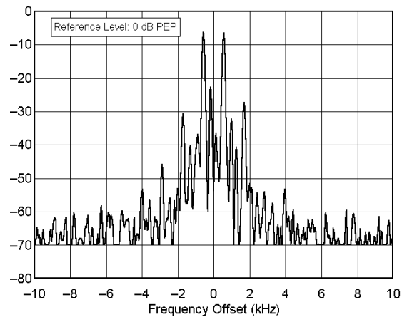
Yaesu FT-847 sn 8C020205 432.200 MHz, Transmit IMD, 50 W F:\SHARED\PROD_REV\TESTS\FT847\FT847170.TXT
