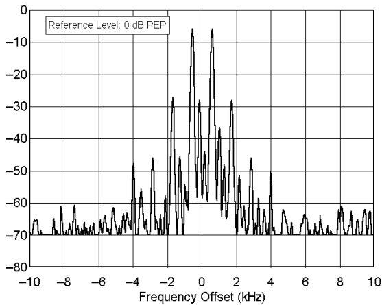
Yaesu FT-847 sn 8C020205 24.950 MHz, Transmit IMD, 100 W F:\SHARED\PROD_REV\TESTS\FT847\FT847112.TXT
