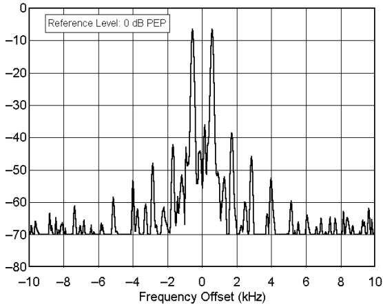
Yaesu FT-847 sn 8C020205 1.850 MHz, Transmit IMD, 100 W F:\SHARED\PROD_REV\TESTS\FT847\FT84710.TXT
