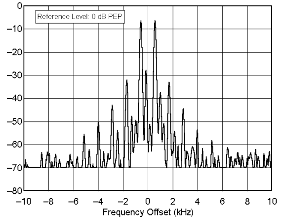
Yaesu FT-847 sn 8C020205 10.120 MHz, Transmit IMD, 100 W F:\SHARED\PROD_REV\TESTS\FT847\FT847100.TXT
