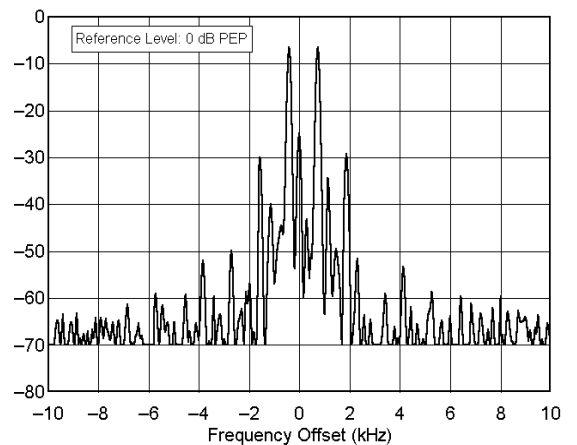
Yaesu FT-847 sn 8C020205 144.200 MHz, Transmit IMD, 50 W F:\SHARED\PROD_REV\TESTS\FT847\FT84712M.TXT
